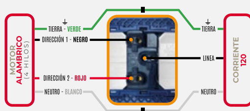
DIAGRAMA DE INSTALACIÓN
